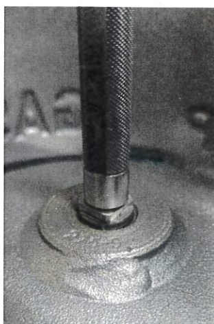
Fot. 2. Wskazanie dla gwintu spełniającego kryterium akceptacji
