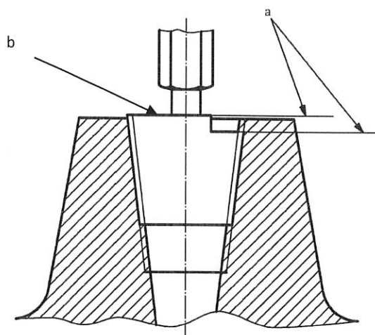
Rys. 2. Sposób kontroli gwintu przy użyciu sprawdzianu trzpieniowego gładkiego:
