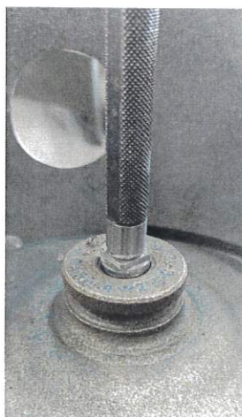
Fot. 1. Sposób zamocowania sprawdzianu w otworze gwintowanym butli
