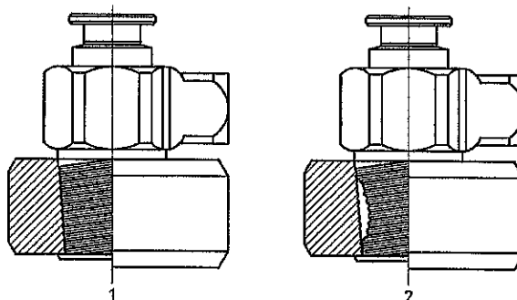
Rys. 3. Taliowanie gwintu na przykładzie trzpienia gwintowanego zaworu butli: 1 - prawidłowy kształt gwintu, 2 - uszkodzona powierzchnia gwintu
